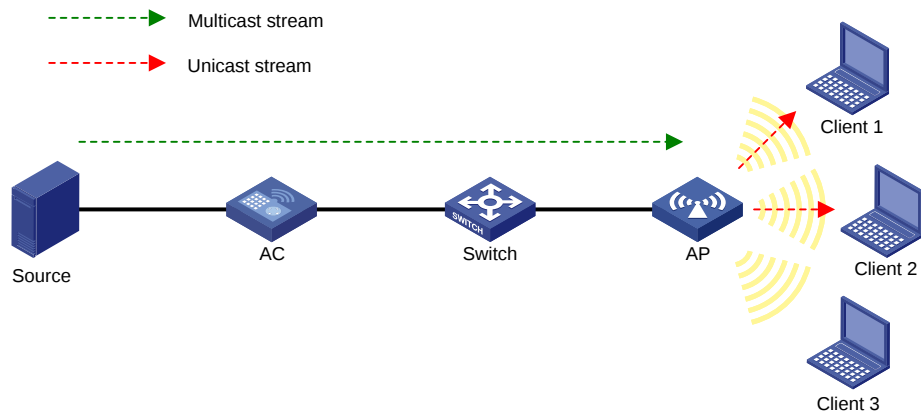
图1-29 组播优化配置组网图
