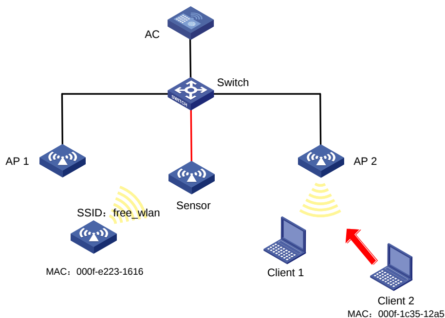
图1-23 WIPS 分类与反制组网图
