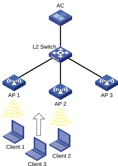
图1-21 带宽模式的负载均衡组网图
