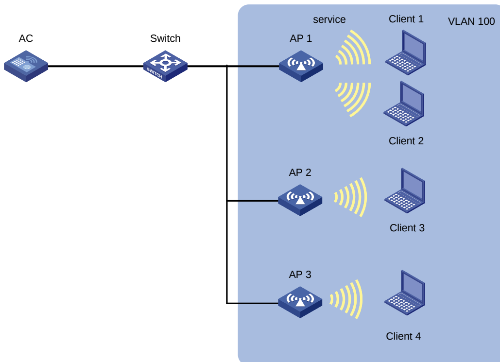
图1-9 指定 AP 的配置文件组网图
