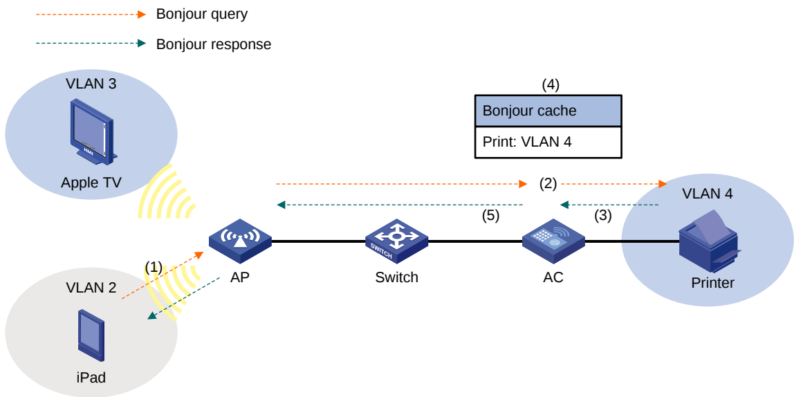
图1-11 Bonjour 网关查询代理过程图
