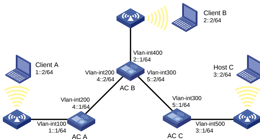
图2-5 IPv6 静态路由配置组网图
