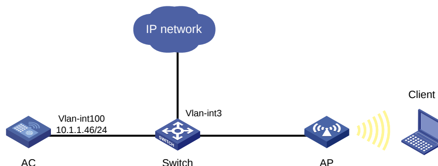
图3-7 支持本地 BYOD 授权的 802.1X 用户认证、授权配置组网图
