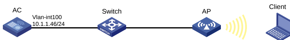
图1-1 共享密钥认证配置组网图
