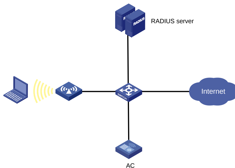
图3-2 802.1X 用户的 RADIUS 认证配置组网图
