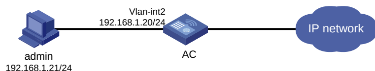
图4-1 管理员配置组网图
