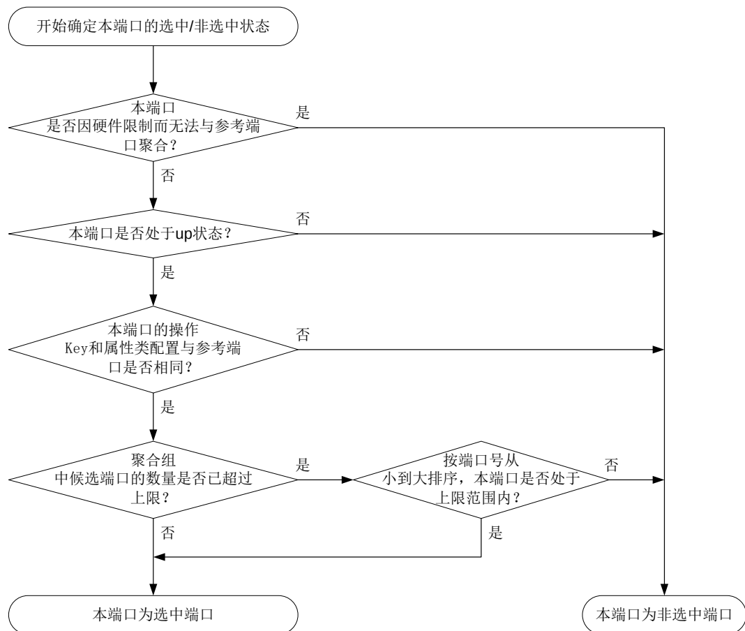
图2-1 静态聚合组内成员端口状态的确定流程
