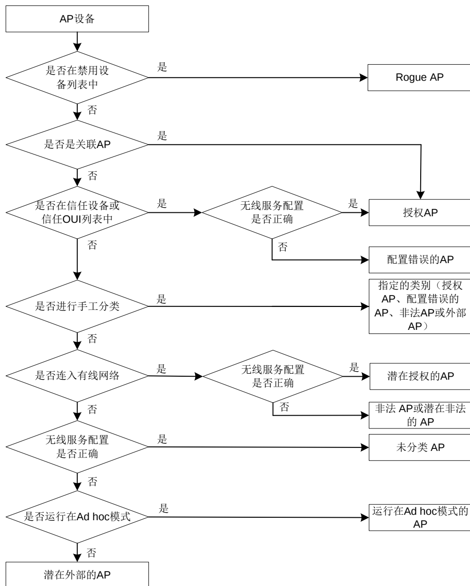
图1-8 WIPS 对检测到的 AP 设备的分类处理流程示意图
