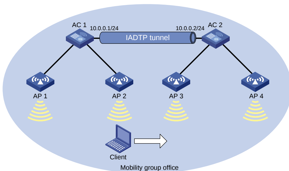
图1-27 AC 间漫游配置组网图
