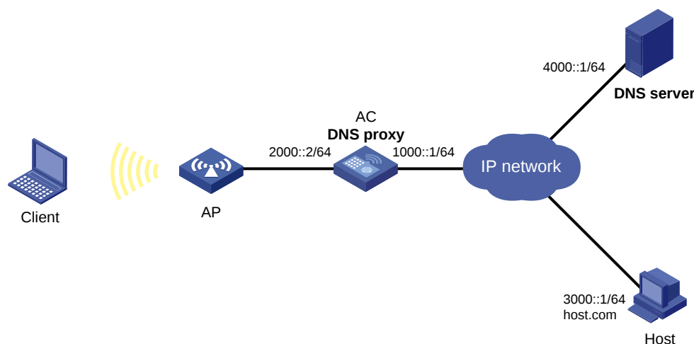
图2-15 IPv6 DNS proxy 配置举例组网图
