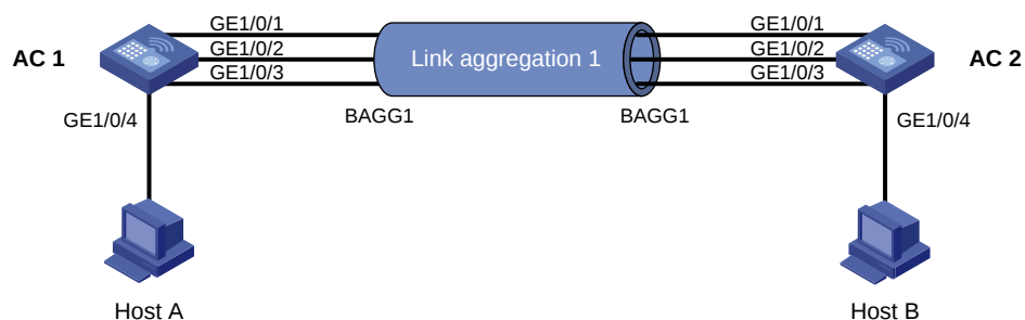
图2-2 以太网链路聚合配置组网图
