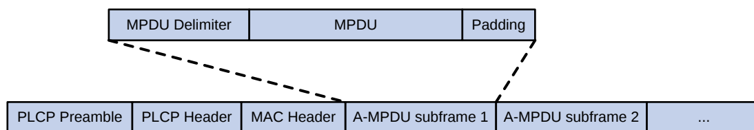
图1-4 A-MPDU 报文格式图
