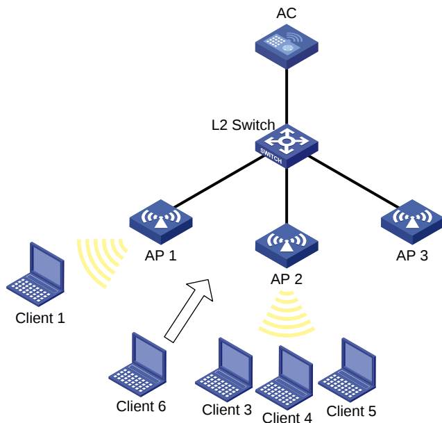
图1-19 会话模式的负载均衡组配置组网图
