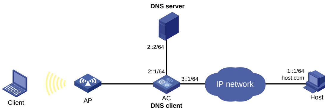
图2-14 动态 IPv6 DNS 配置举例组网图
