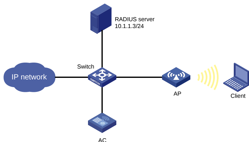
图3-4 802.1X 认证配置组网图
