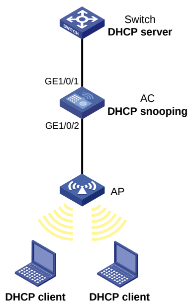
图2-3 DHCP Snooping 配置组网图
