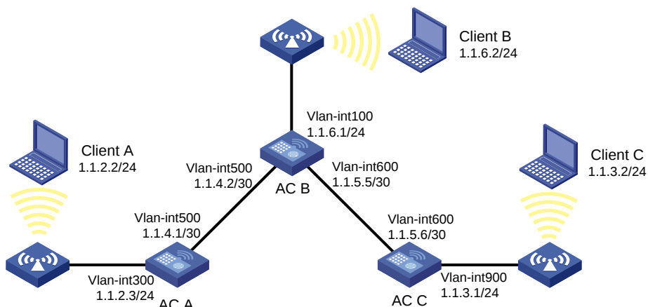
图2-4 IPv4 静态路由配置组网图
