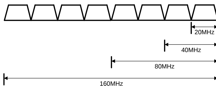
图1-6 802.11ax 信道带宽划定方式示意图
