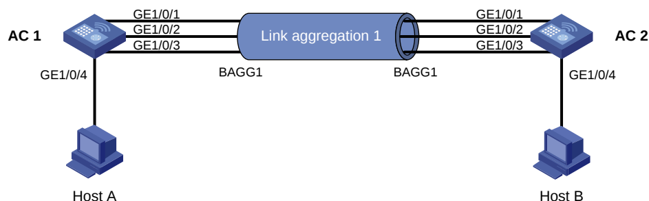
图2-1 以太网链路聚合配置组网图
