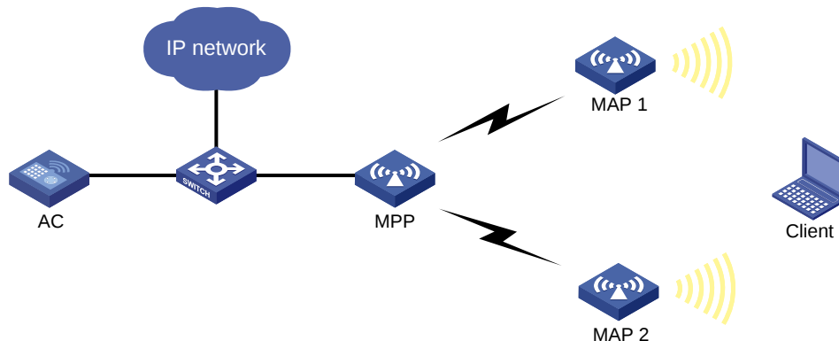
图1-28 集中式 Mesh 网络配置组网图
