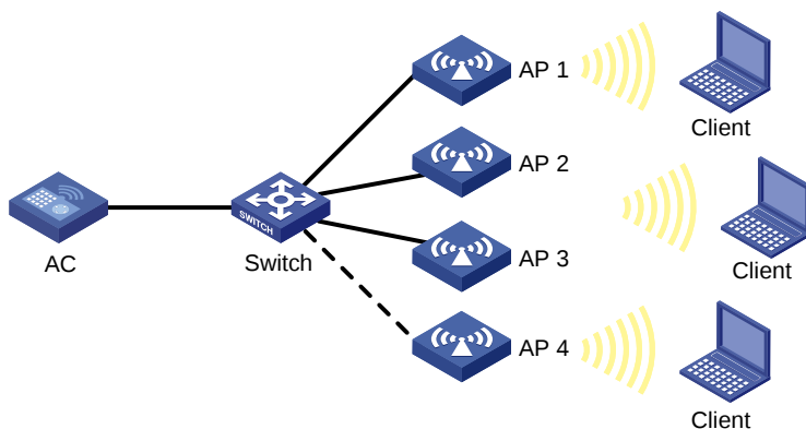
图1-14 自动功率调整配置组网图
