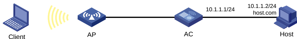
图2-9 静态 IPv4 DNS 配置举例组网图
