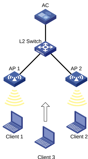
图1-18 带宽模式的负载均衡配置组网图
