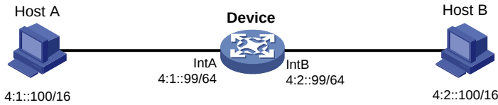
图2-3 普通 ND 代理的典型应用环境
