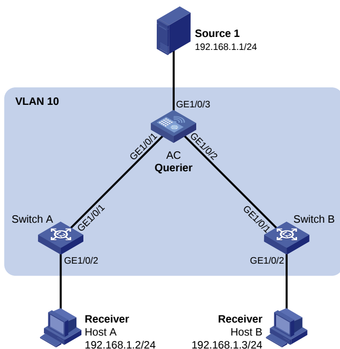
图2-16 IGMP Snooping 配置组网图
