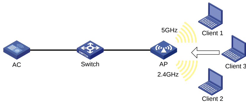
图1-7 启动频谱导航的 WLAN 环境
