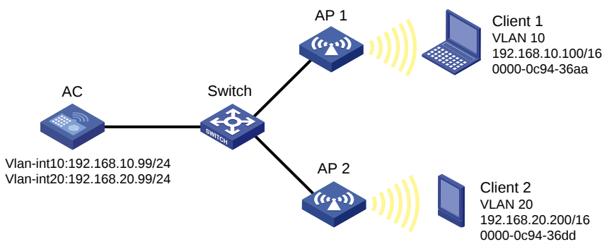
图2-7 代理 ARP 配置组网图
