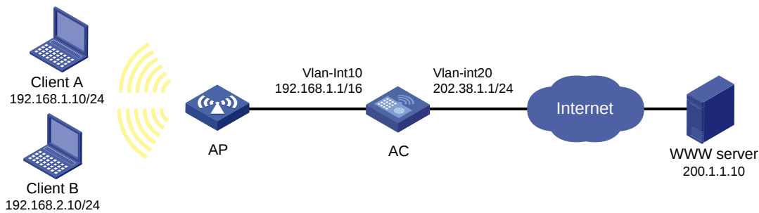
图2-6 内网用户通过 NAT 访问外网
