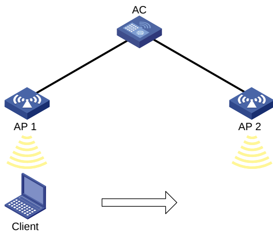
图1-26 AC 内漫游配置组网图
