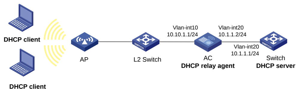
图2-19 组网图
