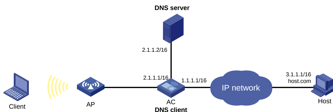
图2-10 动态 IPv4 DNS 配置举例组网图
