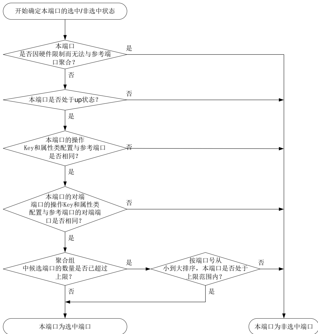
图2-2 动态聚合组内成员端口状态的确定流程
