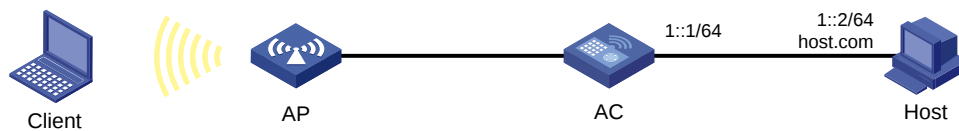
图2-13 静态 IPv6 DNS 配置举例组网图
