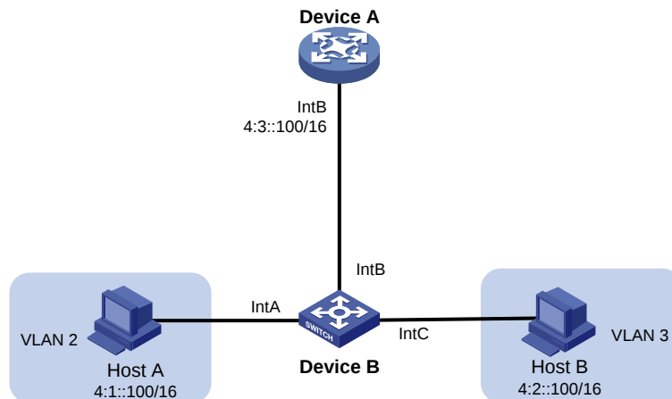
图2-4 本地 ND 代理的应用场景
