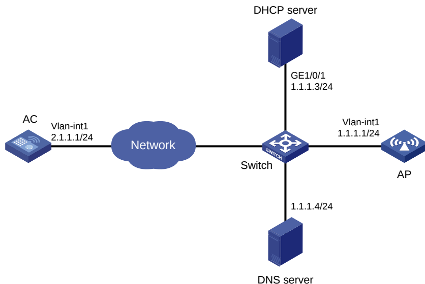
图1-5 通过 DNS 发现方式建立 CAPWAP 隧道典型组网图
