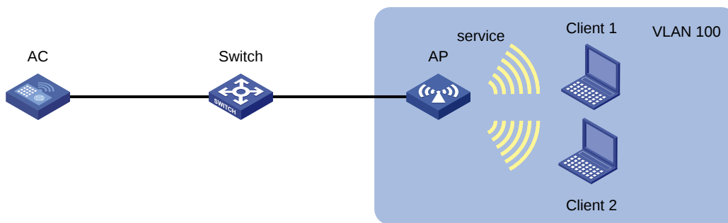
图1-8 指定 AP 的配置文件的组网图
