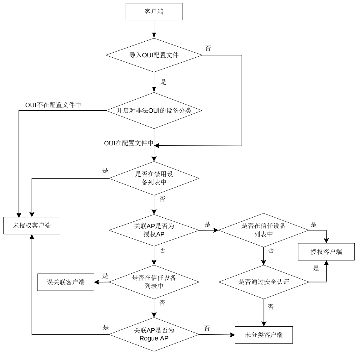
图1-9 WIPS 对检测到的客户端的分类处理流程示意图
