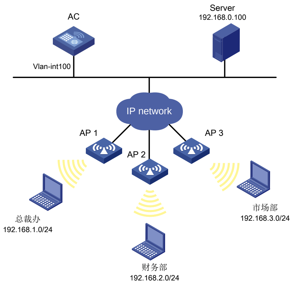
图3-1 通过 ACL 进行包过滤配置组网图
