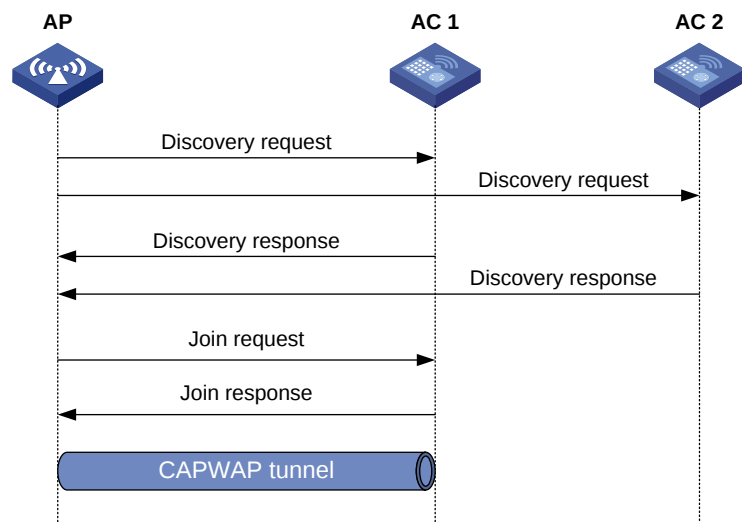
图1-2 CAPWAP 隧道建立过程
