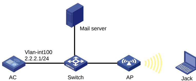
图3-6 来宾用户管理配置组网图
