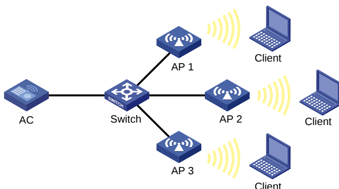
图1-13 自动信道调整配置组网图
