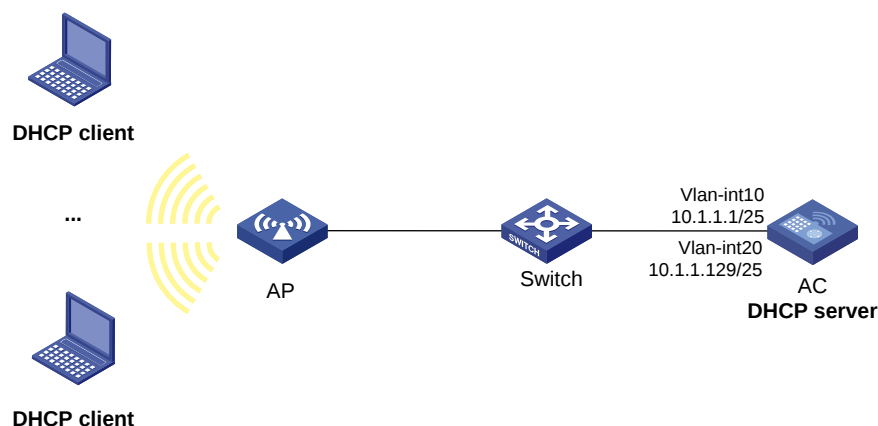
图2-18 DHCP 动态分配地址配置组网图
