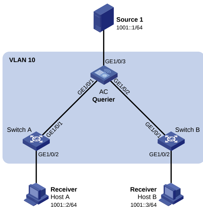
图2-17 MLD Snooping 配置组网图
