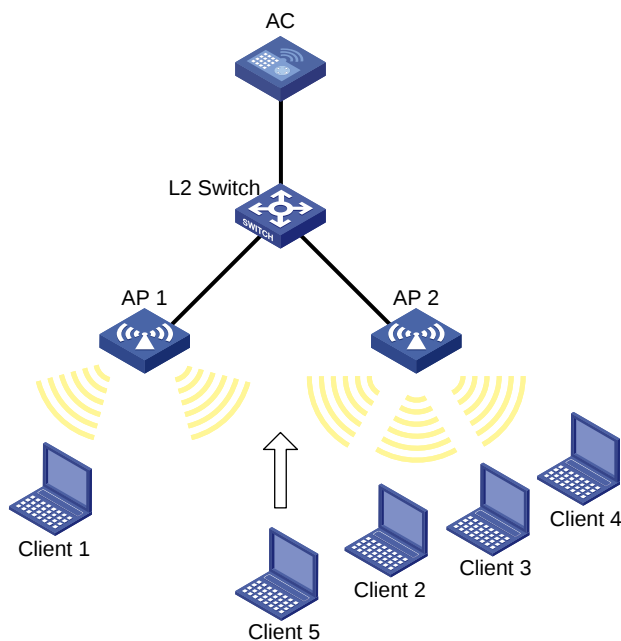
图1-16 会话模式的负载均衡配置组网图
