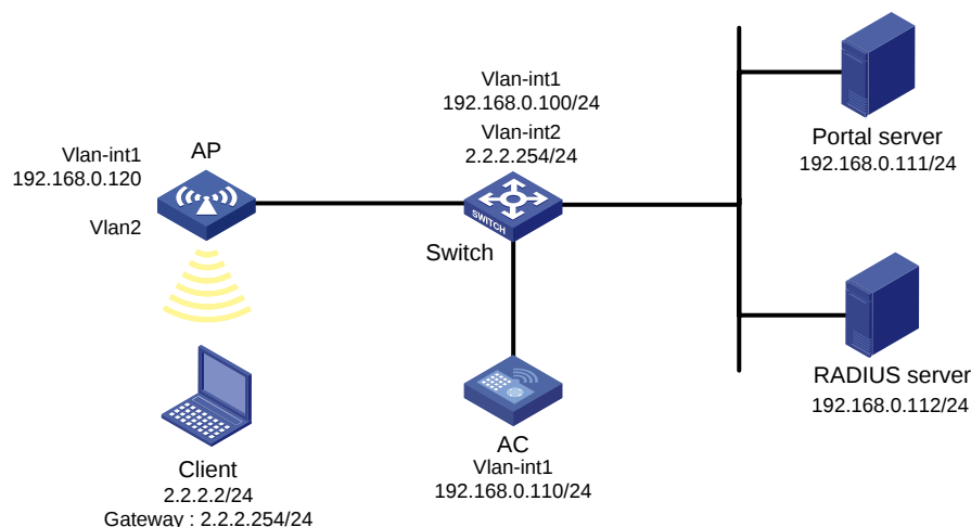
图3-5 Portal 直接认证配置组网图
