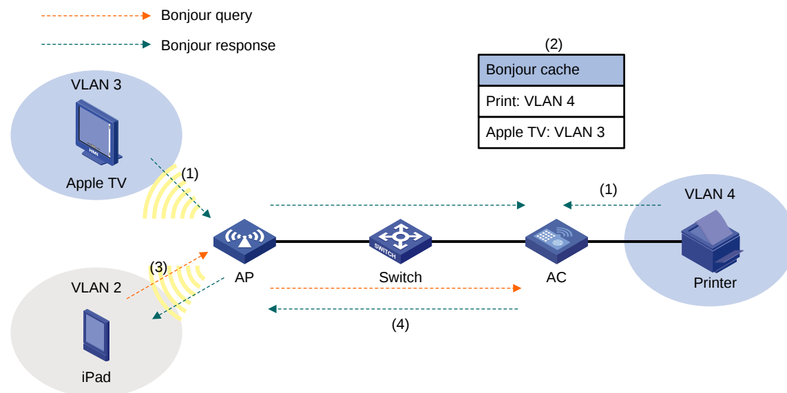
图1-10 Bonjour 网关代答过程图
