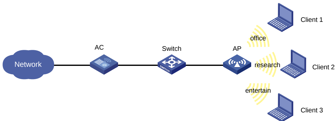
图1-11 智能带宽保障配置举例组网图
