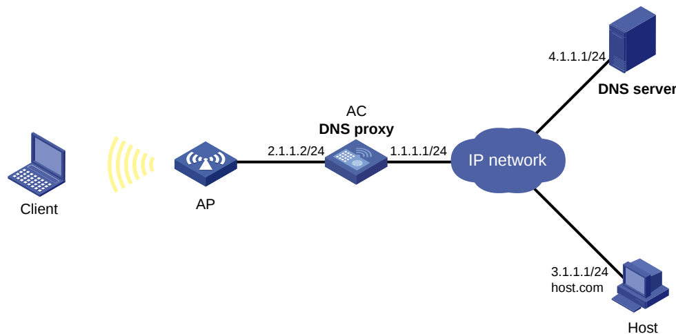
图2-11 IPv4 DNS proxy 配置举例组网图
