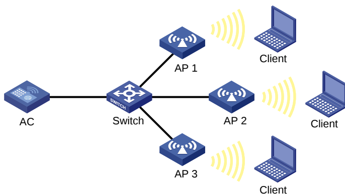
图1-15 自动频宽调整配置组网图
