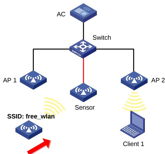
图1-25 WIPS 的攻击检测组网图
