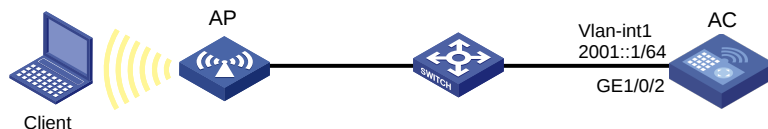
图2-12 IPv6 地址静态配置组网图
