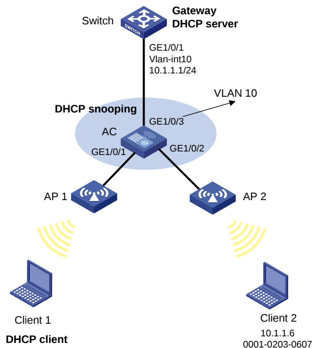
图2-8 配置用户合法性检查和报文有效性检查组网图
