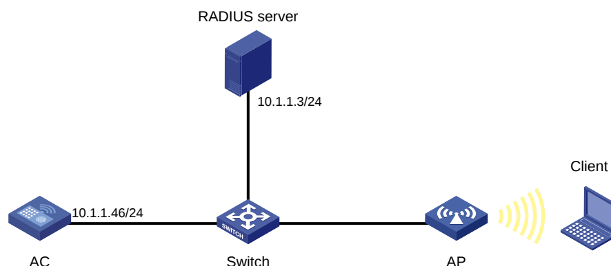
图1-3 PSK 密钥管理模式和 MAC 认证配置组网图
