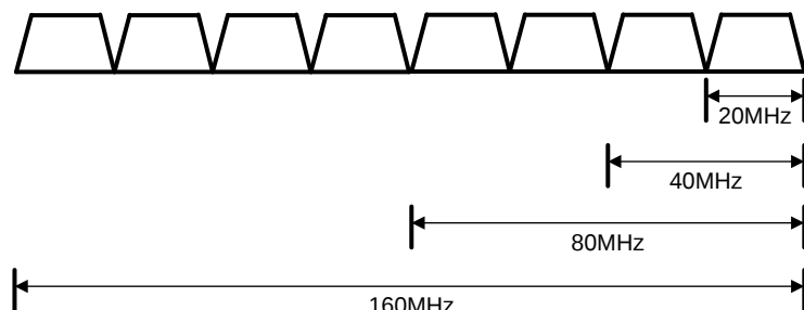
图1-5 802.11ac 信道带宽划定方式示意图
