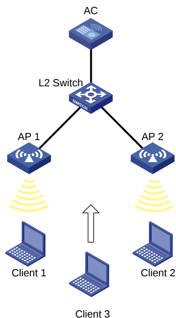
图1-17 流量模式的负载均衡配置组网图
