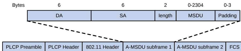
图1-3 A-MSDU 报文格式图
